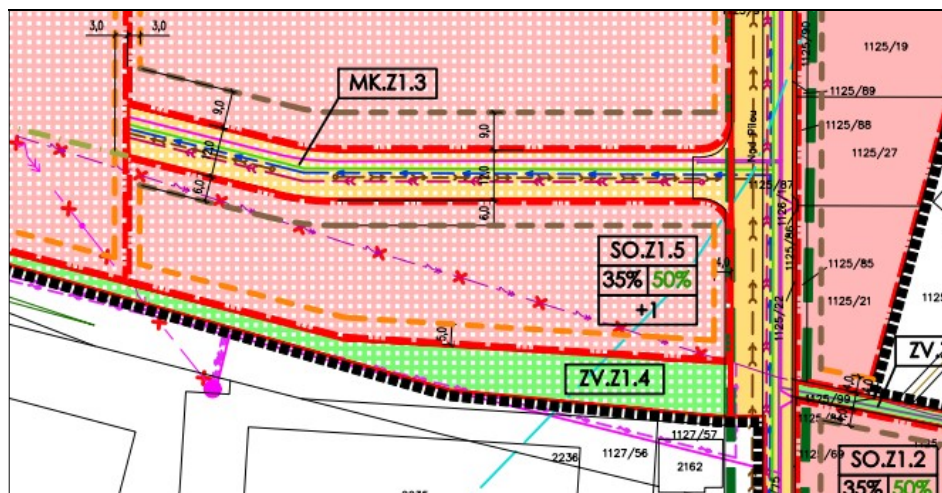
Výřez z RP Hluboká nad Vltavou – lokalita Křesín Pod Pilou – koordinační výkres – ÚZ po změně č.1
